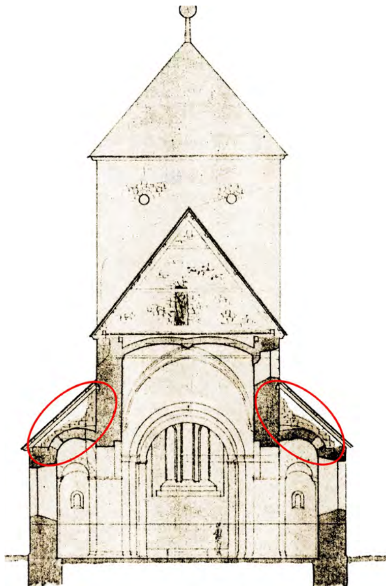
Tvärsektion genom Nicolaikirkan, inmätt år 1901. Notera att det över sidskeppsvalven är inritat två från klerestorieväggarna utskjutande rester efter murar (inringade med rött). Detta är troligtvis rester efter de forna tvärskeppens utskjutande väggar.
